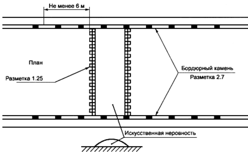
Рисунок 4 - Пример нанесения разметки 1.25 и 2.7 при устройстве ИН
