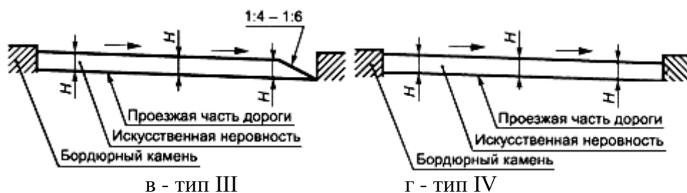
Рисунок 2 - Продольные профили ИН
