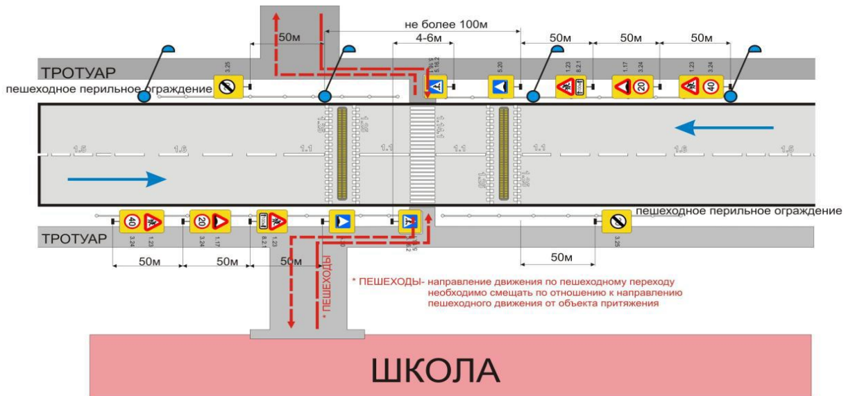
а) ИДН из полимерных материалов
