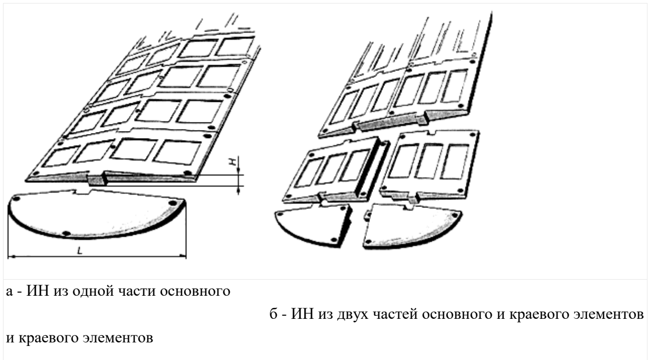
Рисунок 3 - Конструкция сборно-разборной ИН
