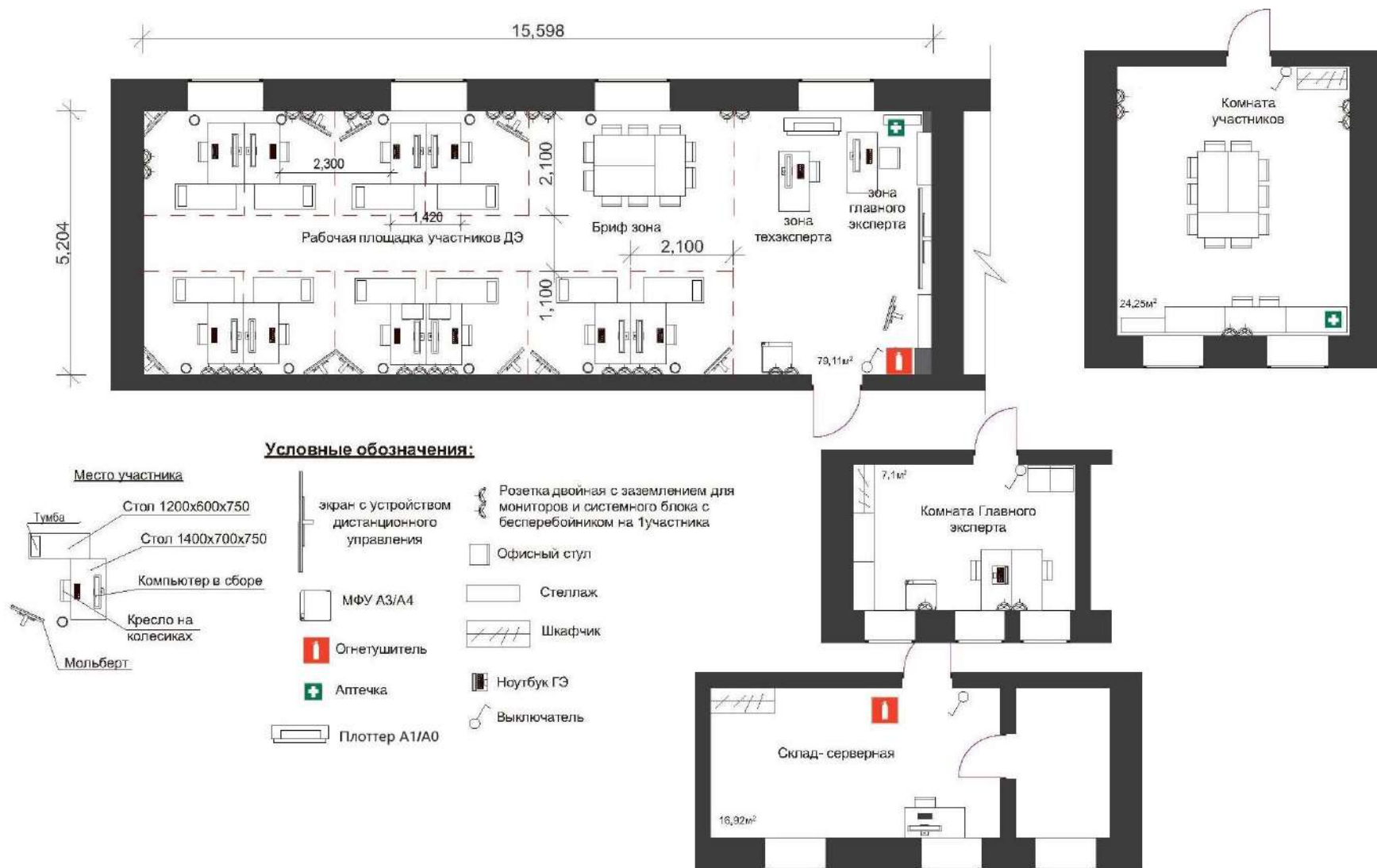
Рисунок VI.2 - План застройки площадки центра проведения демонстрационного экзамена
