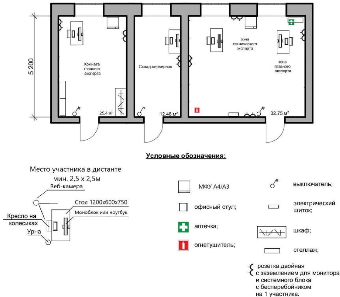
Рисунок III.3 - План застройки площадки центра проведения демонстрационного экзамена
