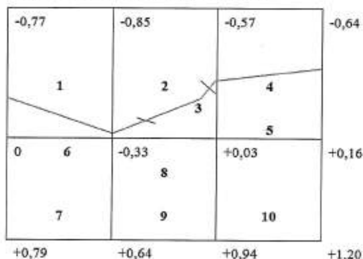
Картограмма земляных работ М 1:500
