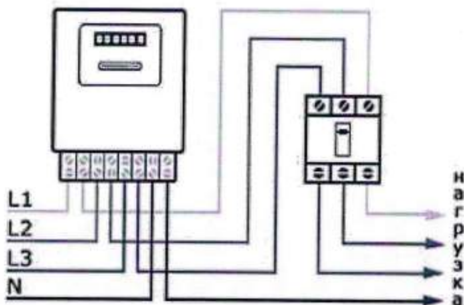
Схема прямого включения трехфазного счетчика
