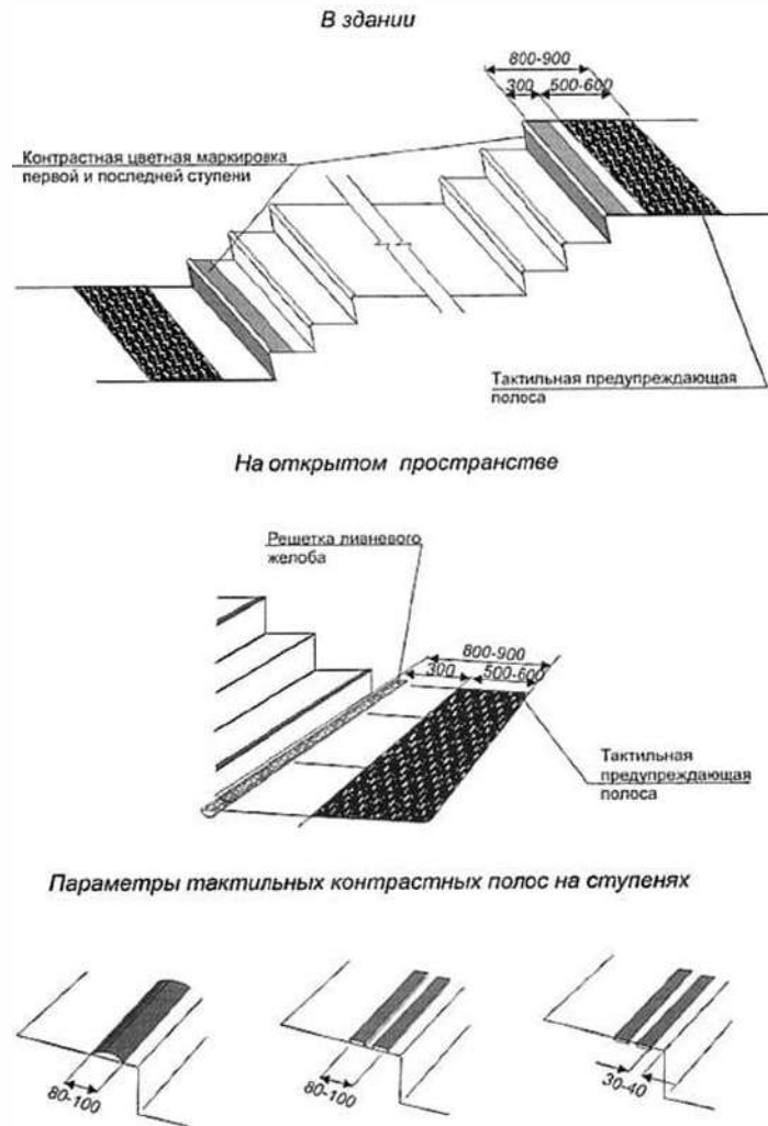
Рисунок В.22 - Предупреждающие контрастные и тактильные полосы
