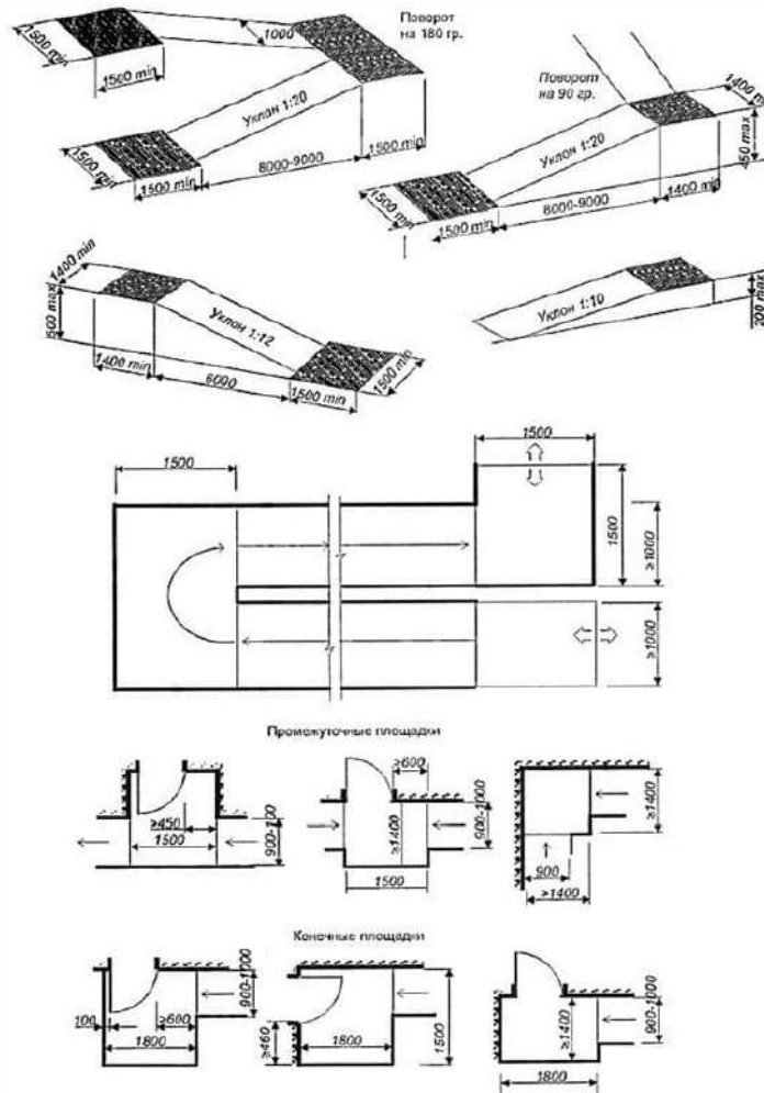
Рисунок В.27 - Площадки пандусов
