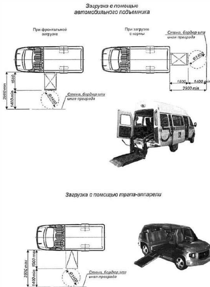
Рисунок В.10 - Параметры зоны посадки-высадки из автотранспорта инвалида на кресле-коляске
