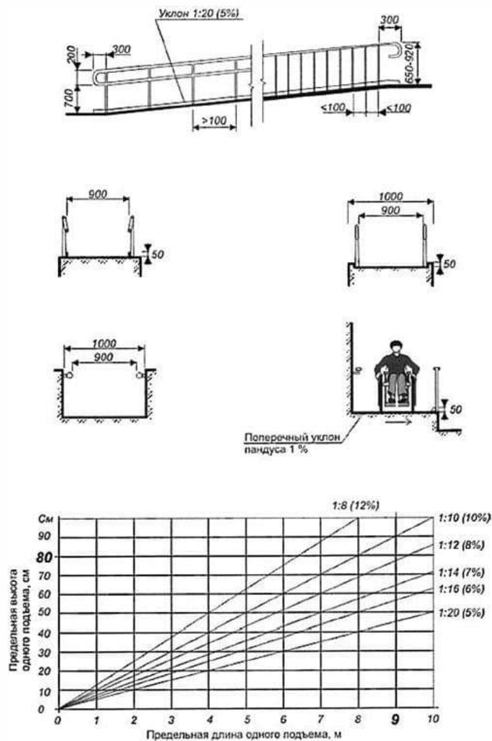
Рисунок В.26 - Основные параметры пандусов
