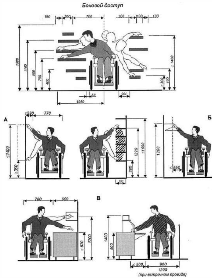
Рисунок Г.3 - Досыгаемость в месте получения услуги
