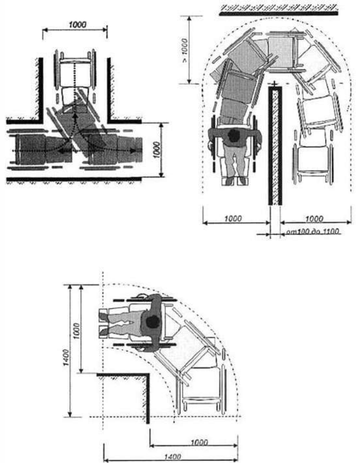
Рисунок В.13 - Размеры поворота и разворота кресла-коляски
