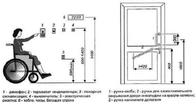
Рисунок Г.6 - Досягаемость оборудования
