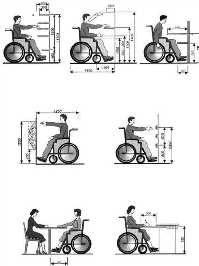
Рисунок Г.2 - Параметры досягаемости в месте получения услуги
