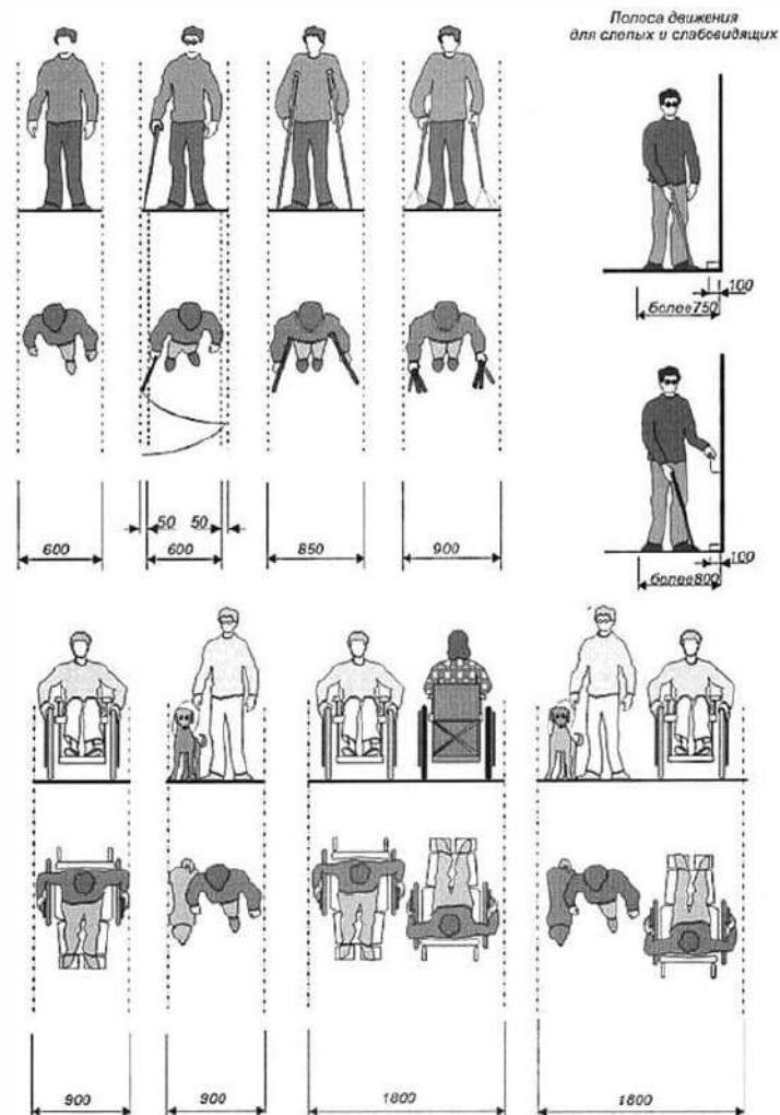
Рисунок В.11 - Габариты полосы движения
