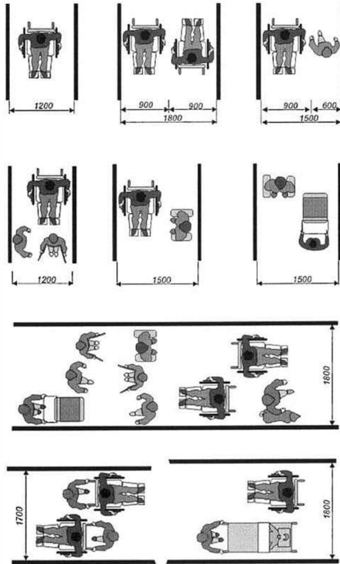
Рисунок В.14 - Параметры и пропускная способность коридоров
