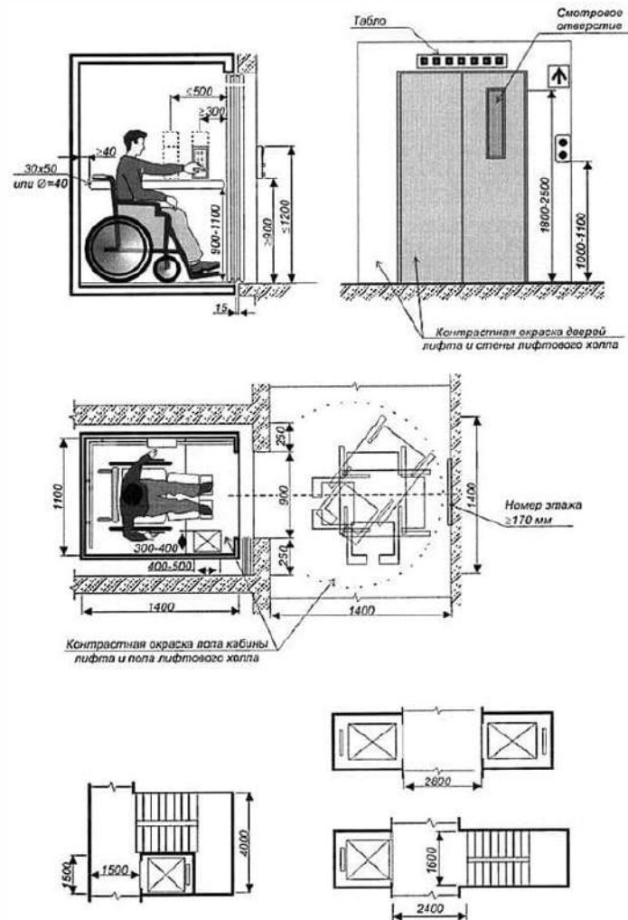
Рисунок В.30 - Габариты лифтов
