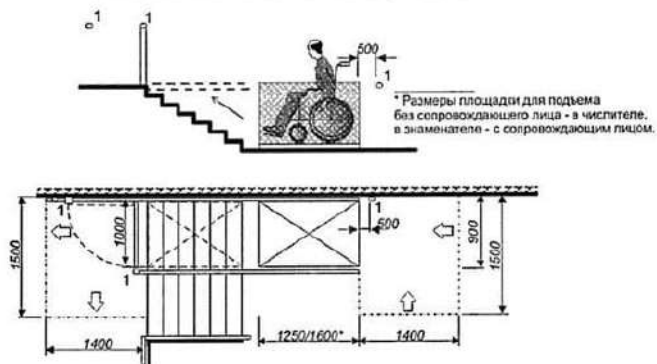
Рисунок В.31 - Параметры наклонных подъемников
