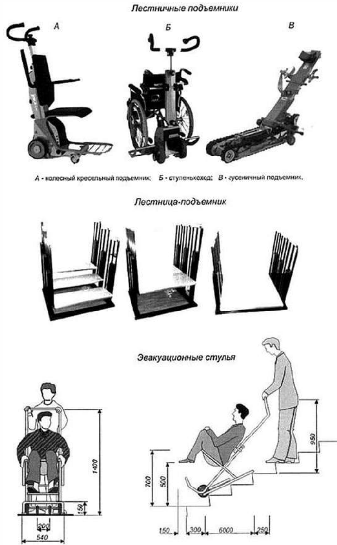
Рисунок В.34 - Автономные транспортные устройства
