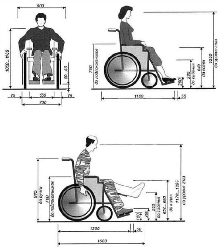
Рисунок В.1 - Габариты кресла-коляски
