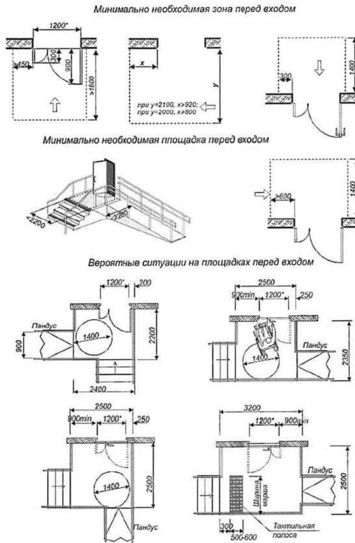
Рисунок В.19 - Площадки перед входами
