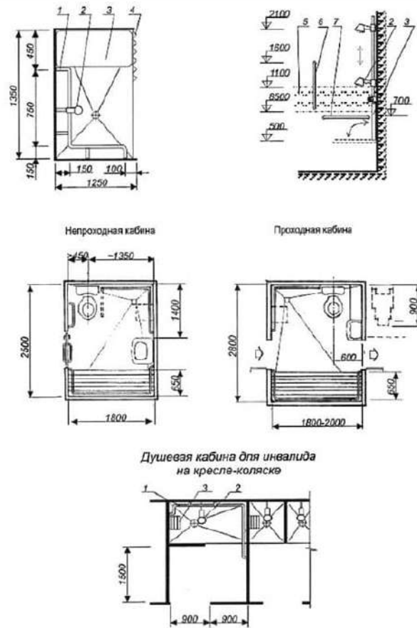
Рисунок Г.11 - Габариты душевых кабин
