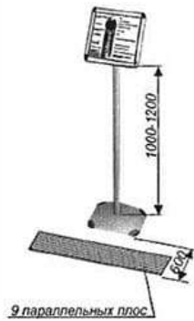
Размещение тактильной полосы перед мнемосхемой
