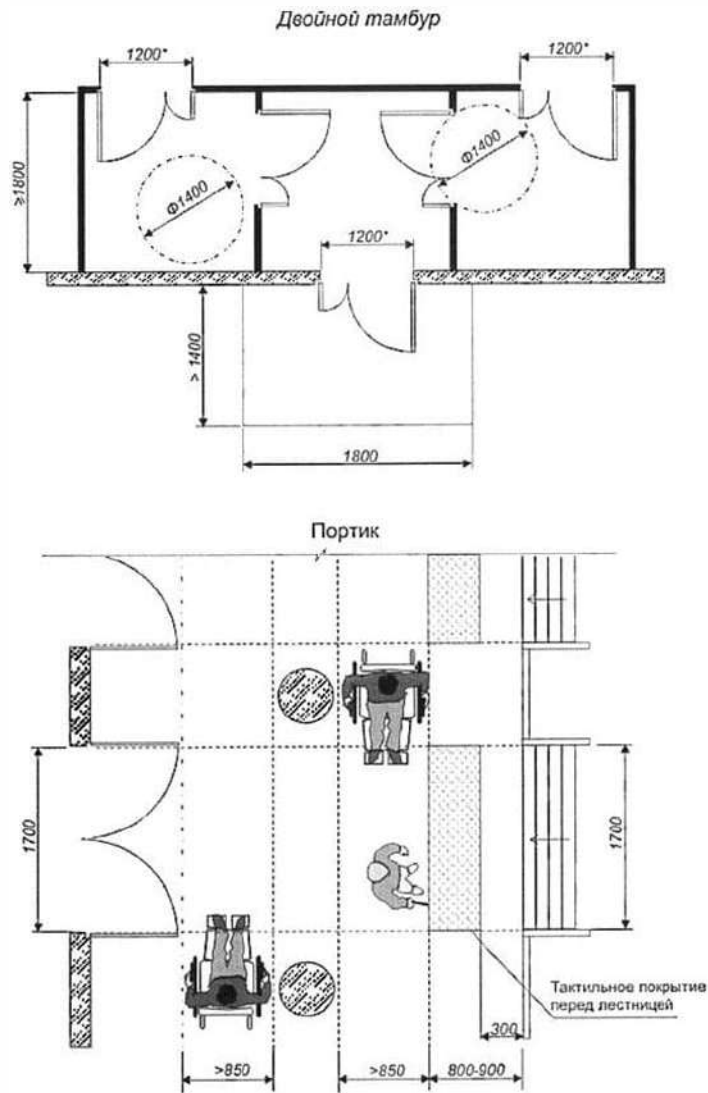
Рисунок В.21 - Площадки перед тамбуром и портиком
