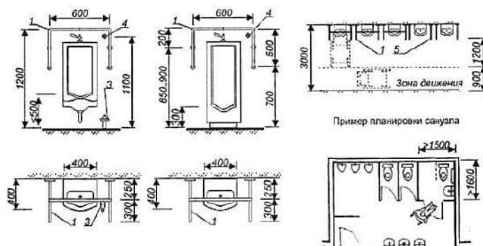
Рисунок Г.8 - Умывальники и писсуары
