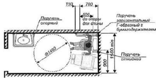
Рисунок Г.12 - Примеры оборудования совмещенного санитарного узла
