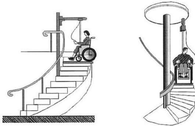
Рисунок В.32 - Индивидуальные подъемные устройства
