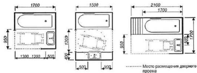
Варианты планировки ванной комнаты
