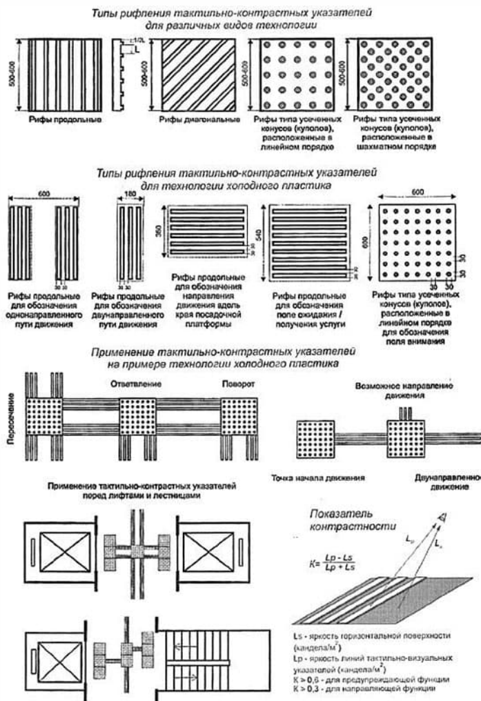
Рисунок Г.18 - Тактильно-контрастные указатели
