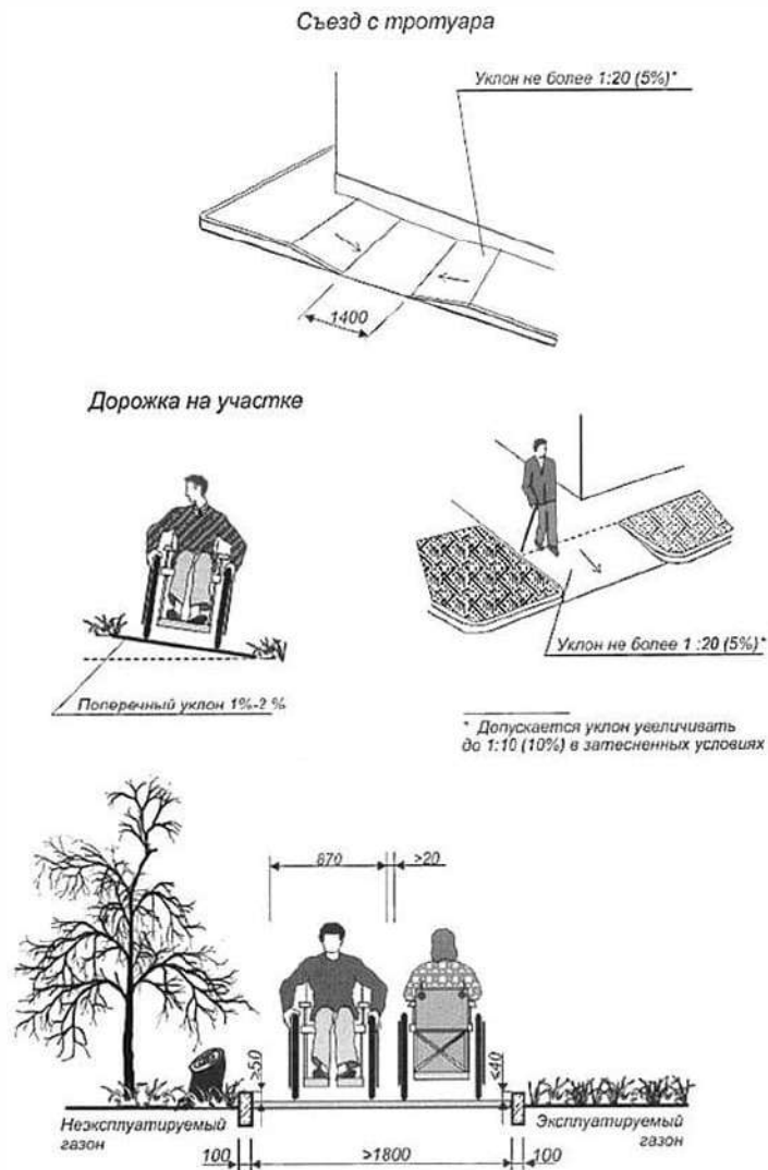
Рисунок В.7 - Организация путей движения на участке
